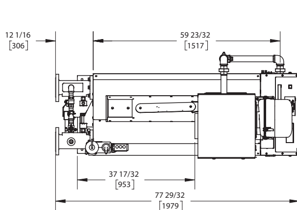
TOP VIEW ASUB-12_F
