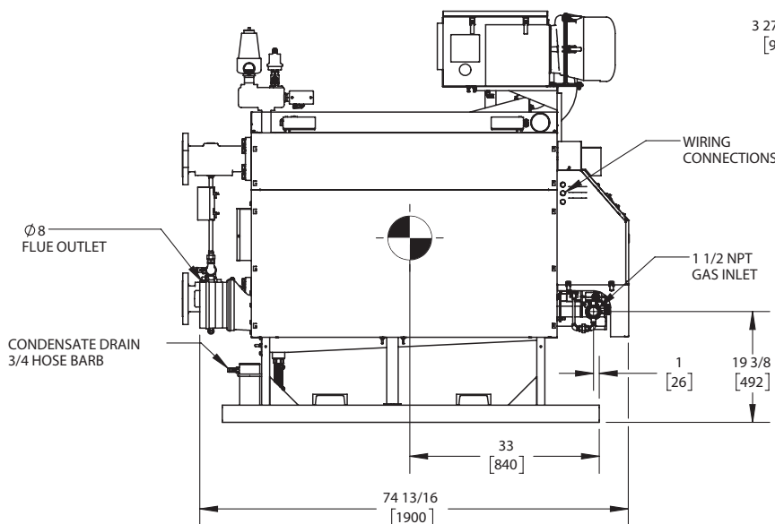
SIDE VIEW ASUB-12_F
